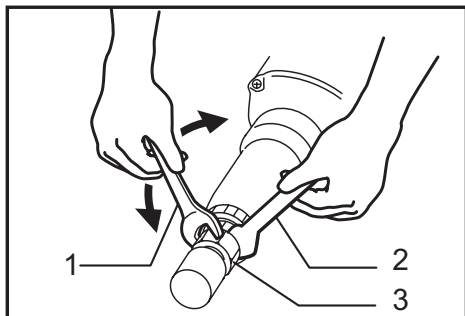
► 1. Clé 19 2. Clé 13 3. Ecrou à collet
